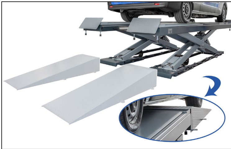
Abbildung: Optionale Auffahrampen TWSA-50U-R
