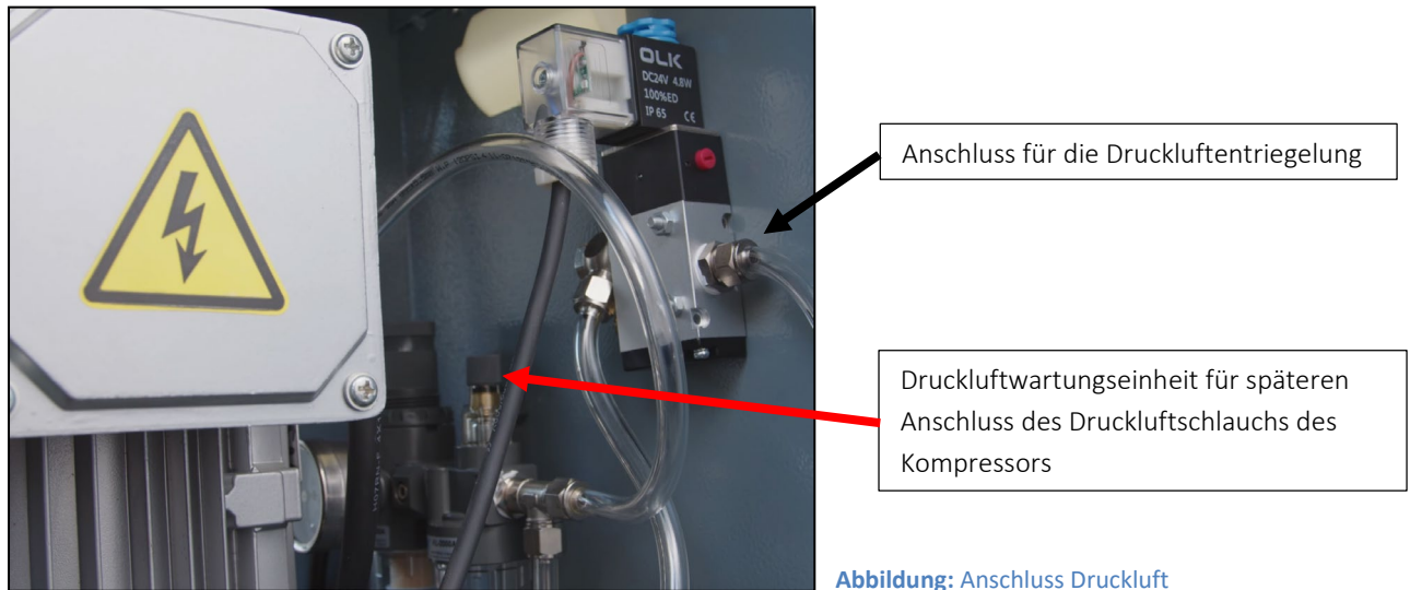
Abbildung: Anschluss Druckluft
